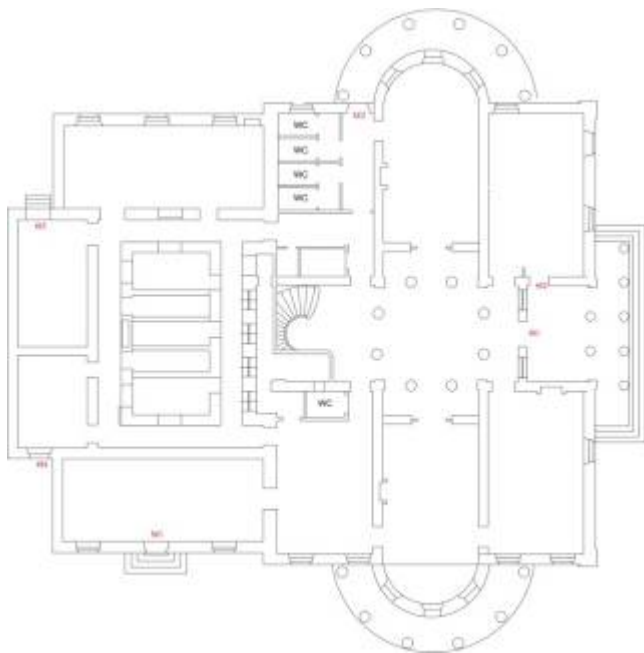
Κάτοψη Ισογείου
